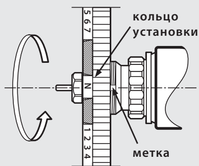
вид "X"
